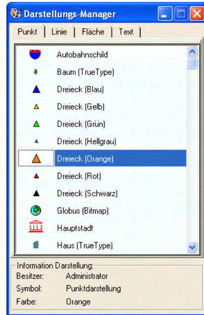
Abbildung 2.46: Der Darstellungs-Manager
