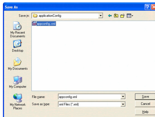
Abbildung 2.52: Konfigurationsdatei speichern
