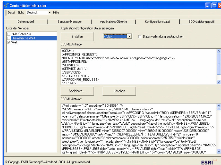
Abbildung 2.51: Konfigurationsdatei erstellen
